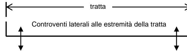
CONTROVENTATURE LATERALI MINIME IN TRATTA
